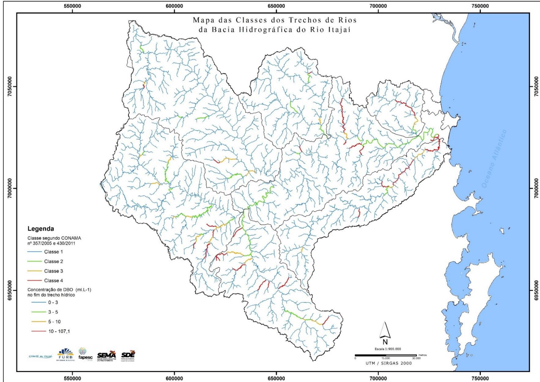
Figura 15 – Cenário atual (2017) dos rios da BHRI em relação ao parâmetro DBO_{5,20^{\circ}C}(Q_{98})
