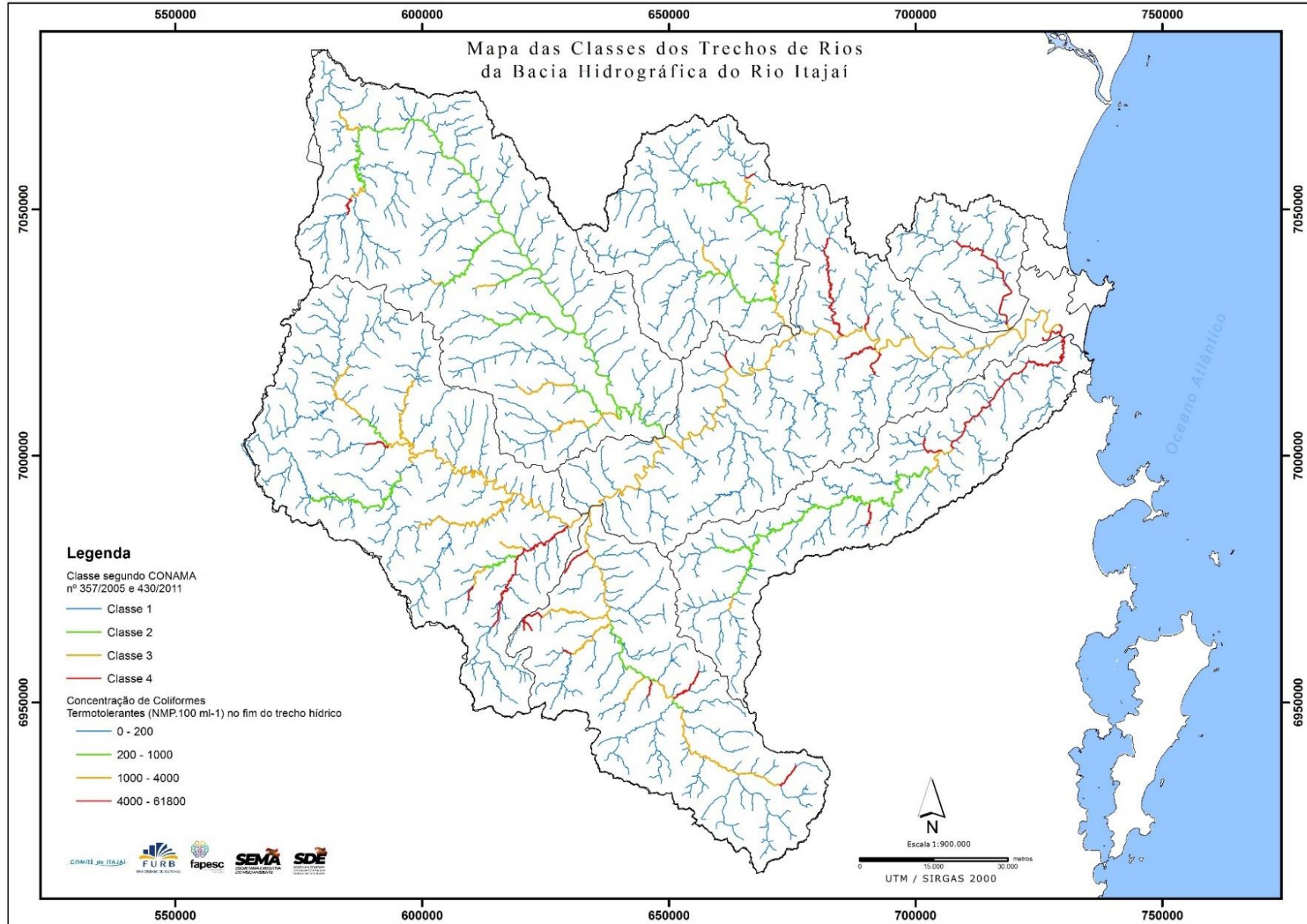
Figura 16–Cenário atual (2017) dos rios da BHRI em relação ao parâmetro Coliforme Termotolerante ( Q_{98\%} )
