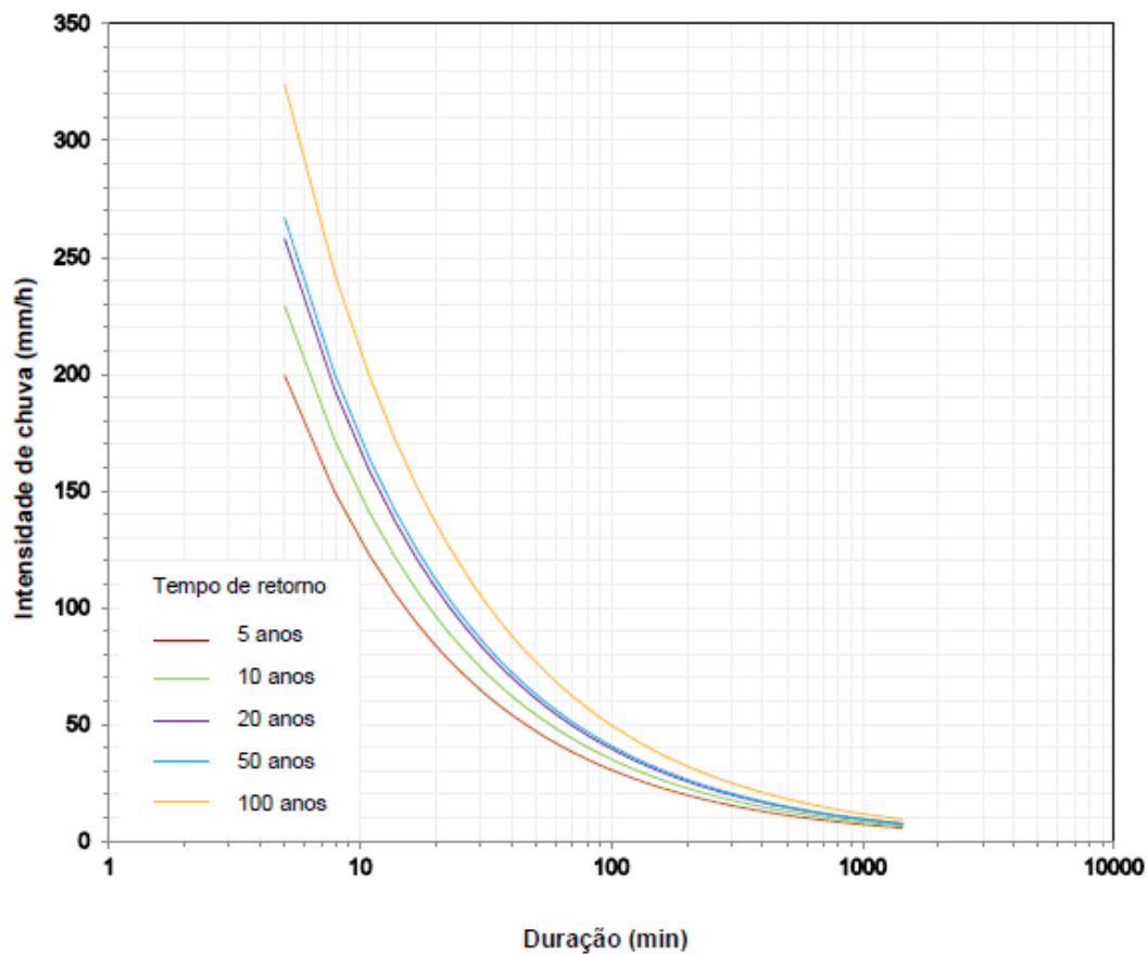
Figura 14- Curva I-D-F para a RH7
