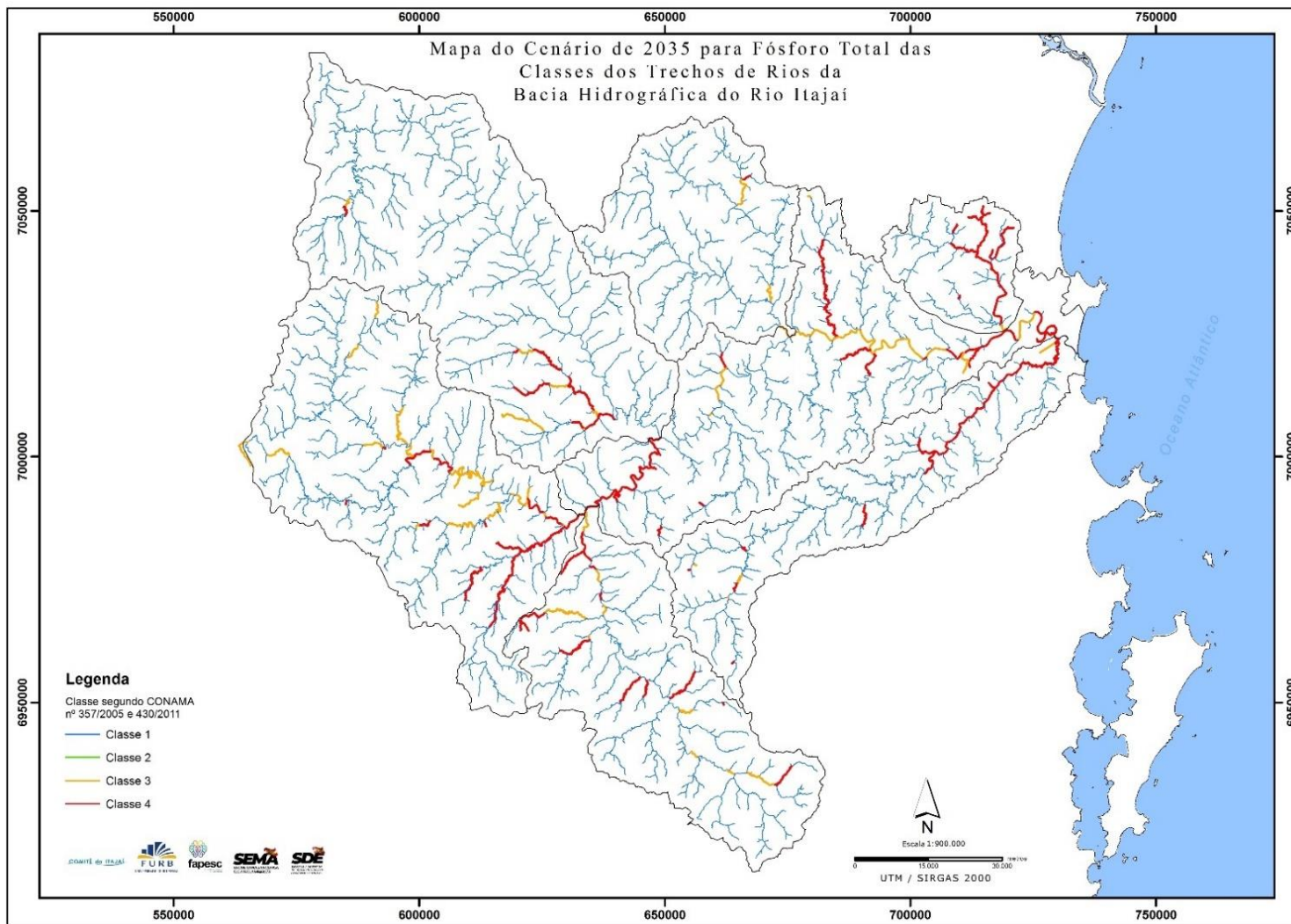
Figura 45- Classe dos rios em relação ao parâmetro fósforo total em 2035 com eficiência nos tratamentos de 60% e 50% da população atendida, Q_{98\%} .
