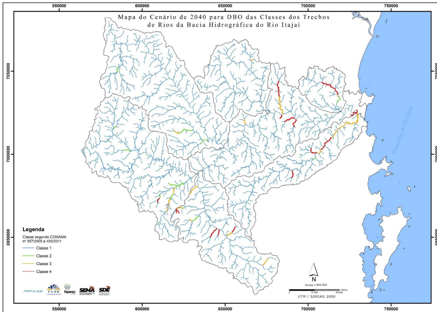
Figura 46 – Classe dos rios para DBO_{5,20^{\circ}C} em 2040, eficiência nos tratamentos de 80% e 80% da população atendida, Q_{98\%}
