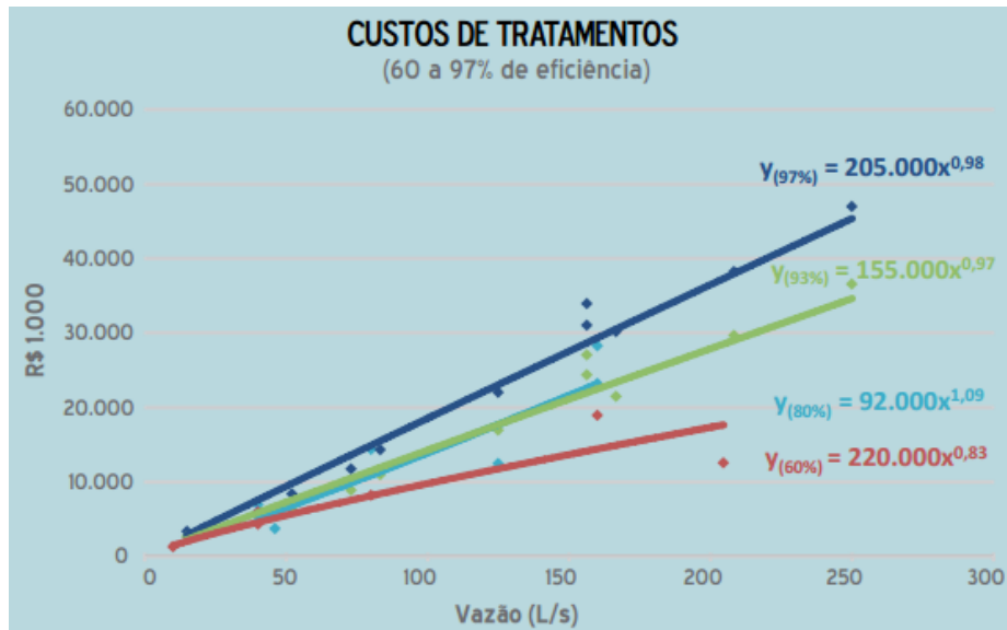
Figura 33 - Custos de Sistemas de tratamentos de efluentes com eficiência de 60 a 97%
