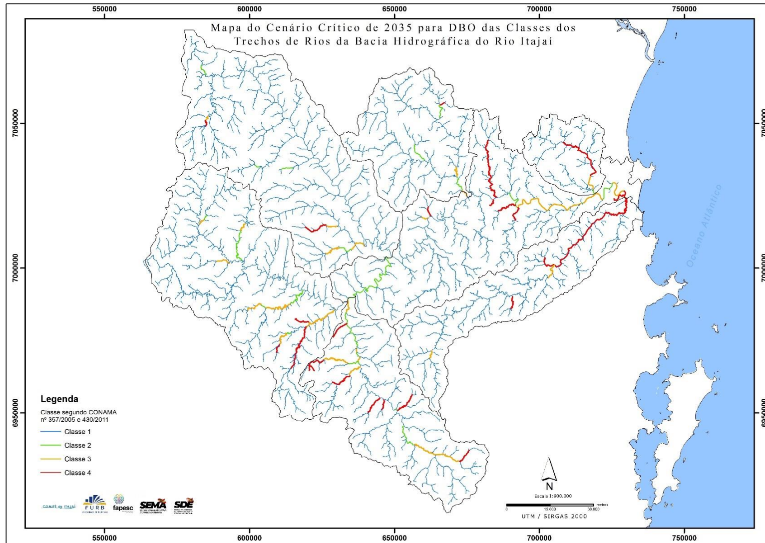
Figura 66 – Classe dos rios em relação ao parâmetro DBO_{5,20^{\circ}C} em 2035, cenário crítico, Q_{98\%}
