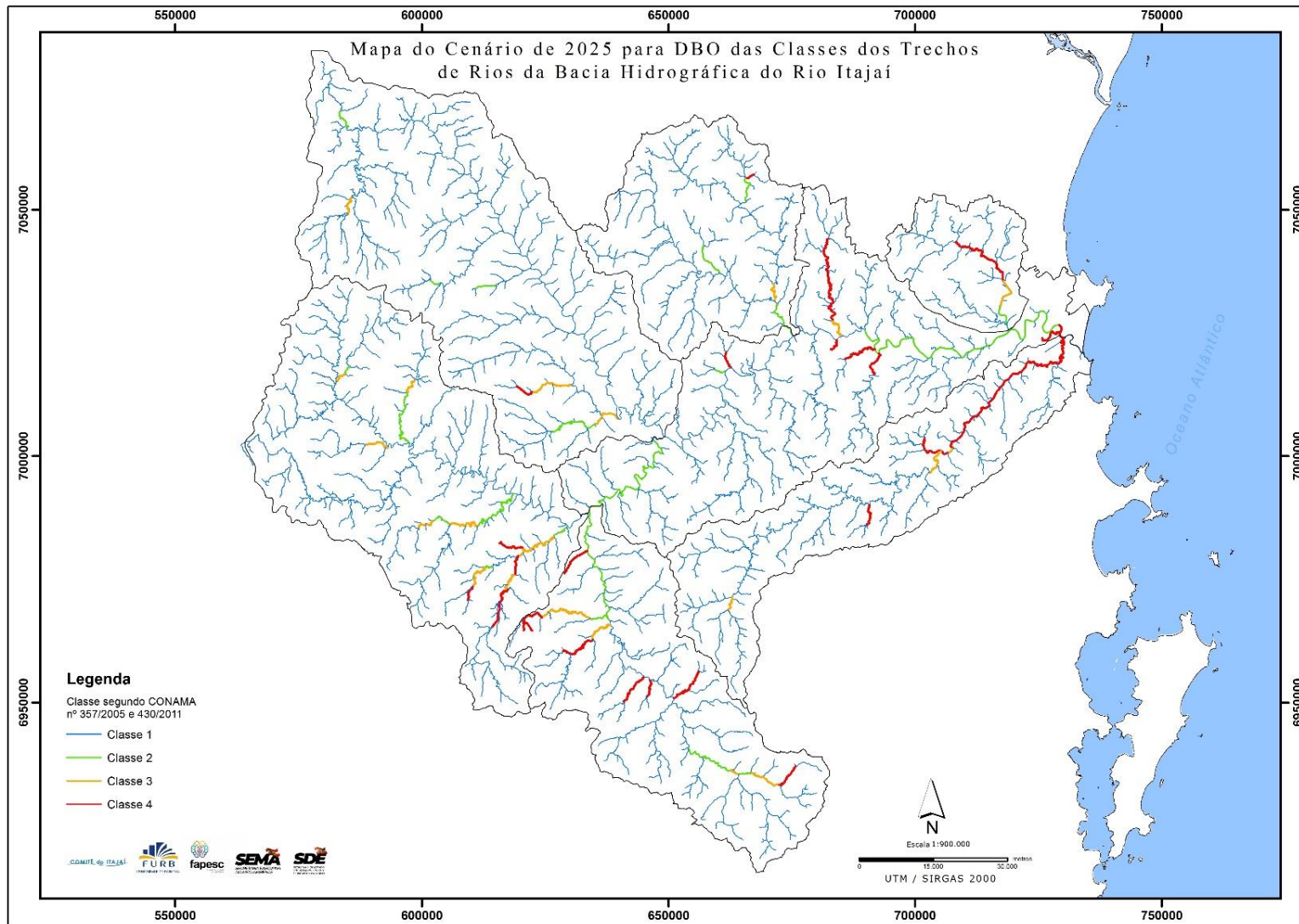
Figura 64- Classe dos rios em relação ao parâmetro DBO_{5,20^{\circ}C} em 2025, com eficiência nos tratamentos de 80% e 15% da população atendida, Q_{98\%}
