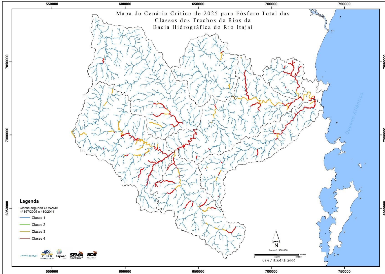
Figura 70 – Classe dos rios em relação ao parâmetro fósforo total em 2025, cenário crítico, Q_{98\%}
