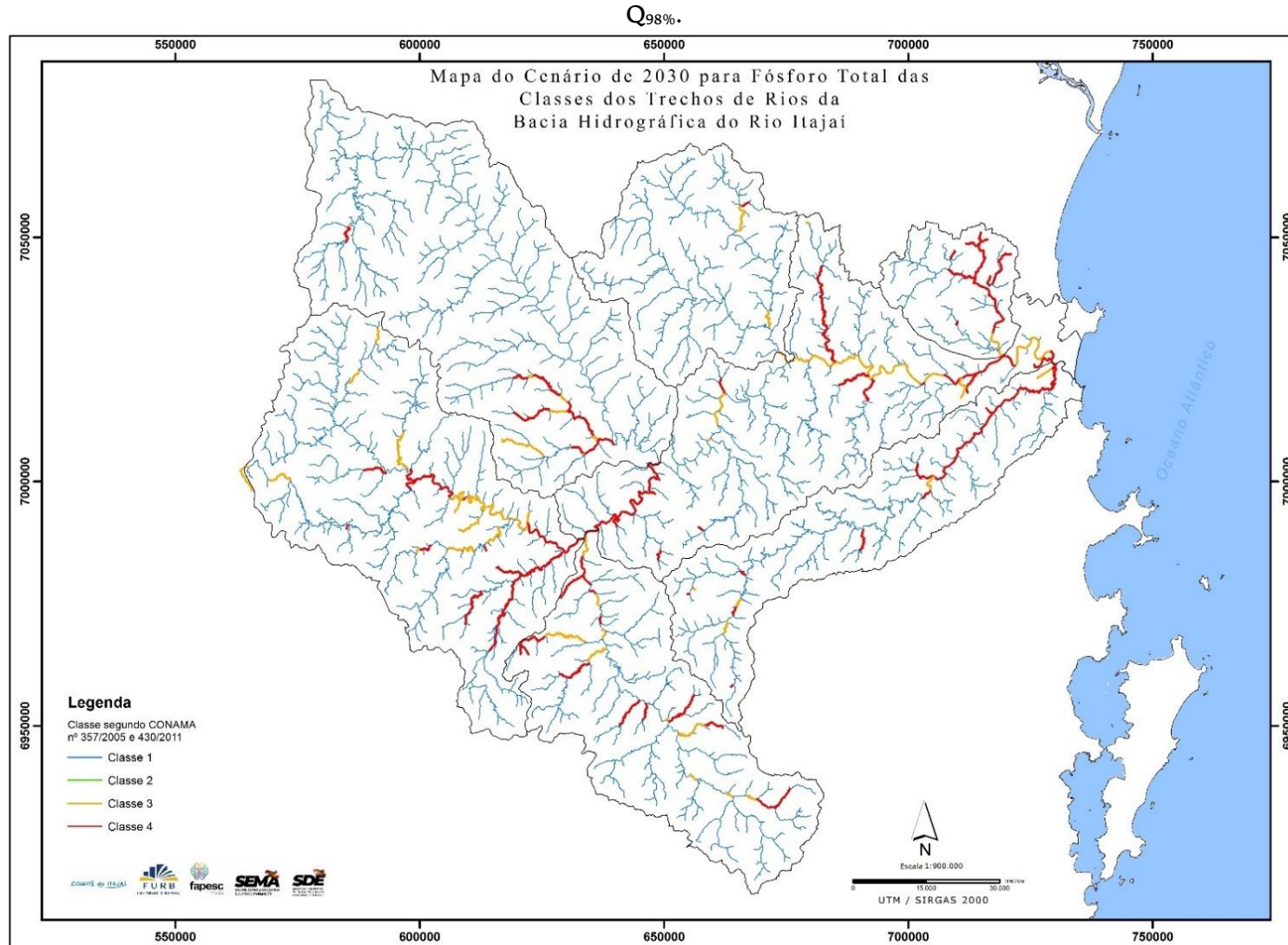
Figura 42 – Classe dos rios em relação ao parâmetro fósforo total em 2030 com eficiência nos tratamentos de 60% e 30% da população atendida,
